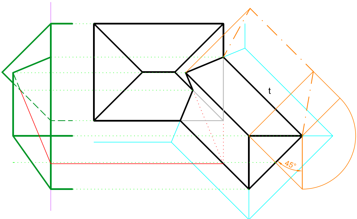
Walmdach mit schräg anlaufendem Nebendach:
