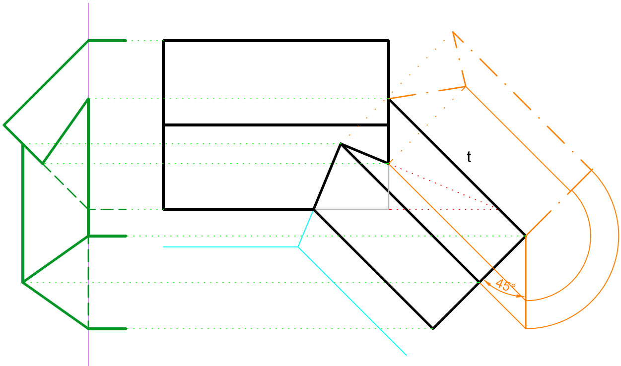
Satteldach mit schräg anlaufendem Nebendach:
